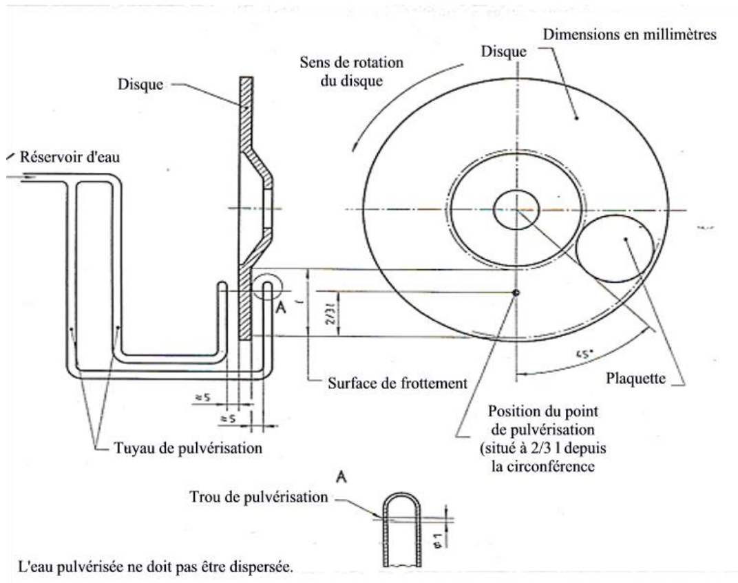
figure 3 : Équipement de pulvérisation d'eau sur frein à disque
